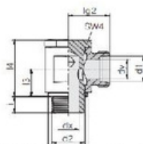
WH - Metri
