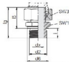
EGE - BSP
