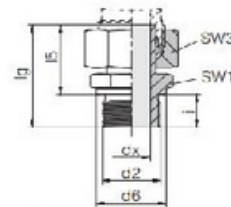
EGE - Metri
